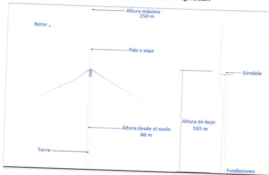
Figura 1-12. Esquema componentes de un aerogenerador.
